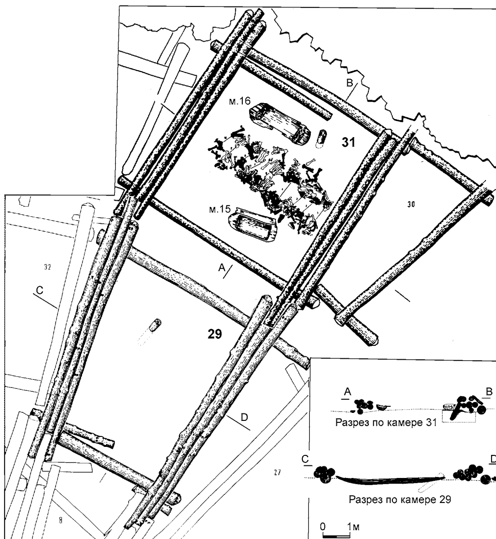
Рис. 1. Кургan Аржан. План и разрезы камер 29 и 31 из Научного архива ИИМК РАН
